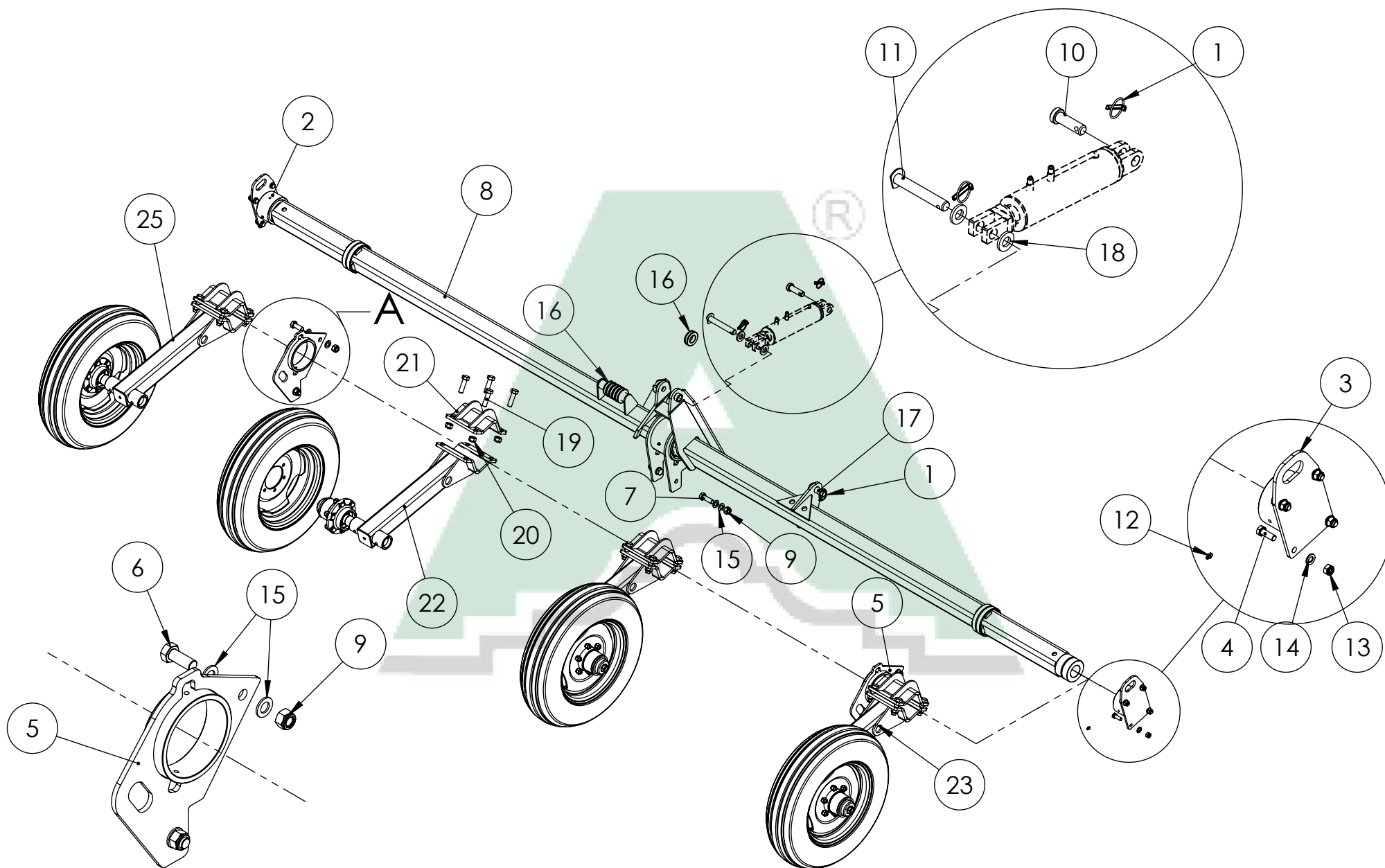
Detalhe A
